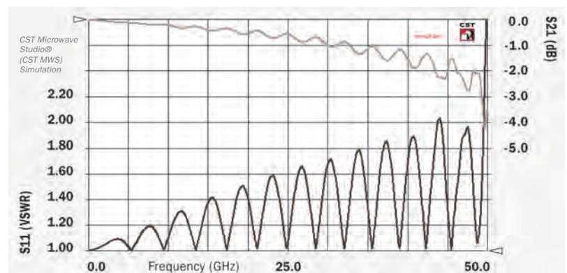
Taper (version 1)
